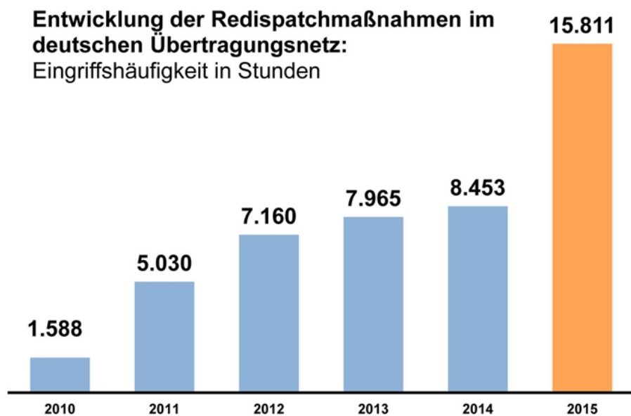
Bild 8: Eingriffshäufigkeit im deutschen Übertragungsnetz
