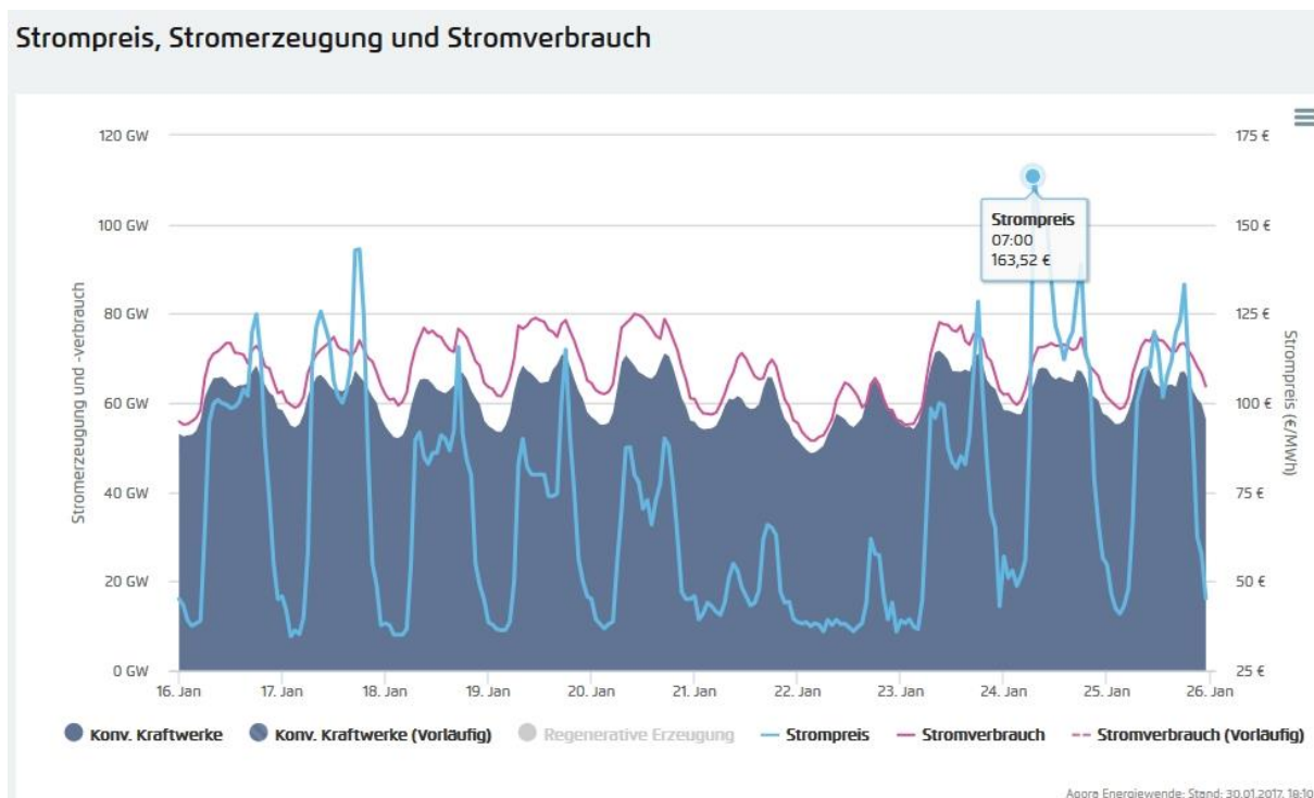
Bild 5: Korrelation Stromverbrauch, Erzeugung der konventionellen Anlagen und Strombörse in Leipzig im Zeitraum 16. bis 26. Januar 2017 (Quelle: Agora)
