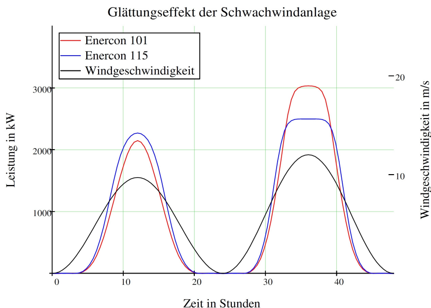
Abbildung 2: Anstieg und Abfall von Windgeschwindigkeit und Leistung
