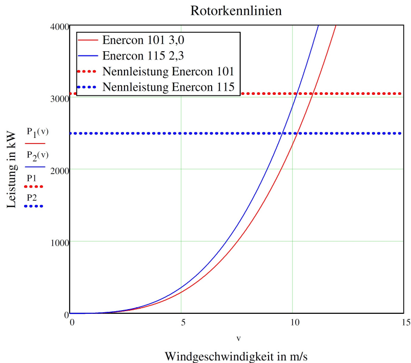
Abbildung 1: Kennlinien und Abregelung der Rotorkennlinien von Enercon 101 und Enercon 115
