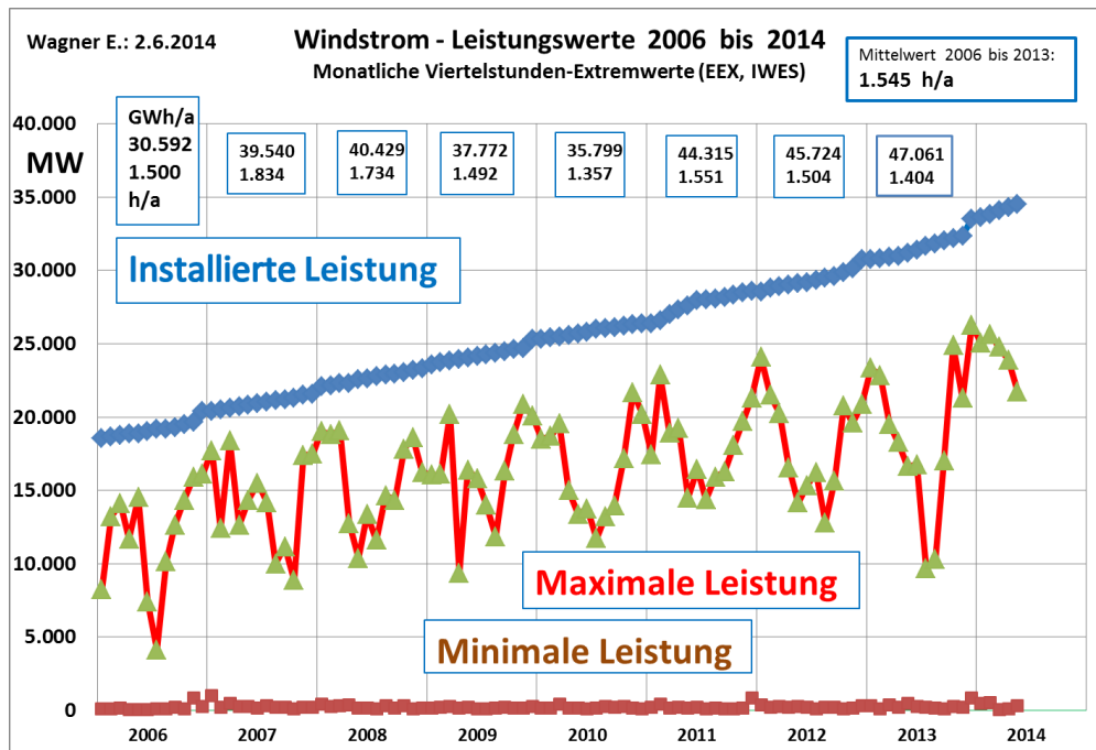
Bild 2: Windstrom-Leistungswerte 2006 bis 2013 monatliche Viertel-Stunden-Extremwerte auf Basis der Strombörse Leipzig (EEX, IWET) Quelle: Eberhard Wagner, Bensheim (2013).
