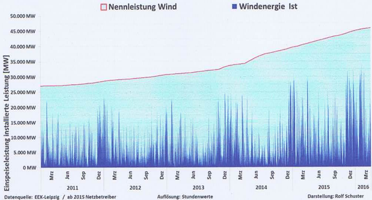
Abb. 1: Windkraftkapazität versus Stromerzeugung
