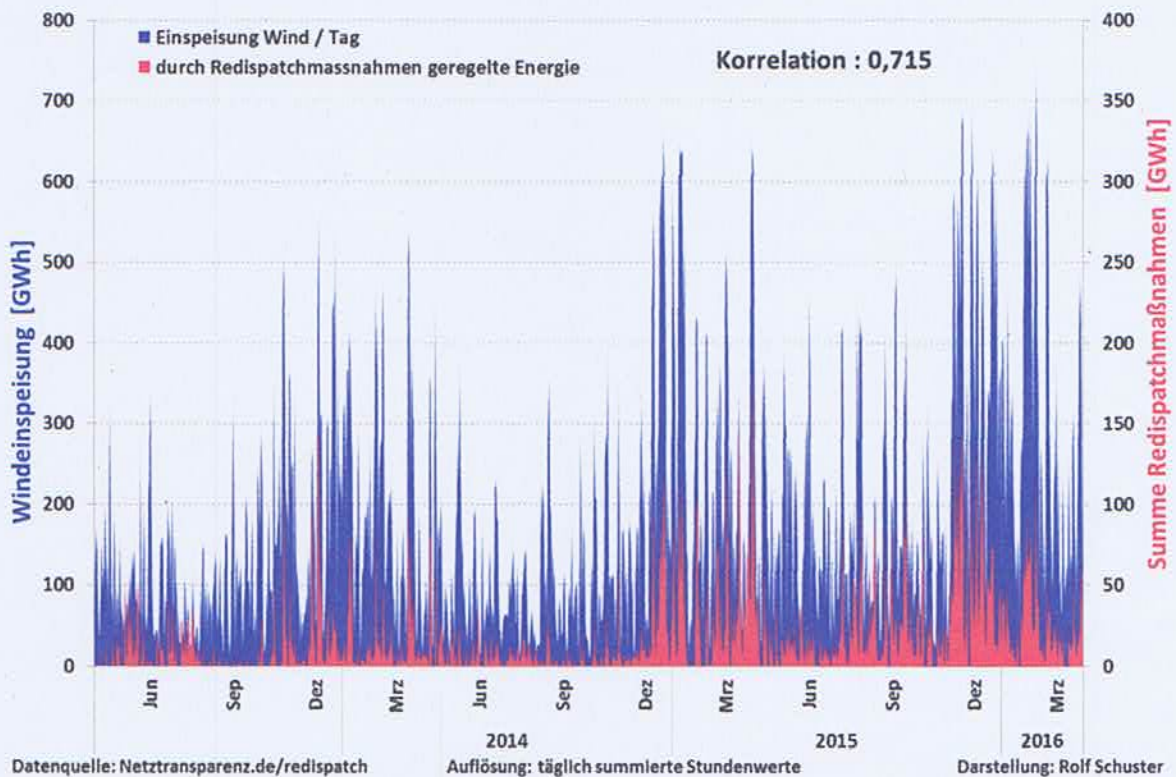
Abb. 3: Windstromerzeugung und Redispatchmaßnahmen
