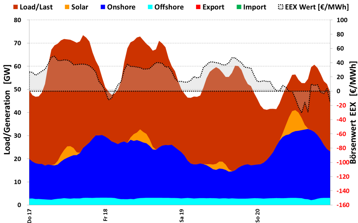
Bild 6: Stromverbrauch und Lastganglinien der Windenergie- und Photovoltaikanlagen im Zeitraum 17. bis 20. November 2016
