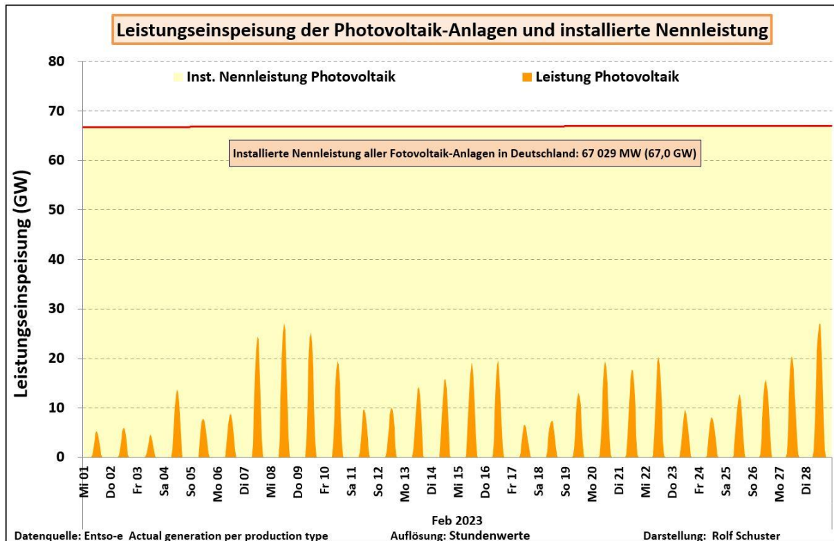
Abb. 2: Leistungsganglinie der Photovoltaik-Anlagen in Deutschland im Februar 2023
