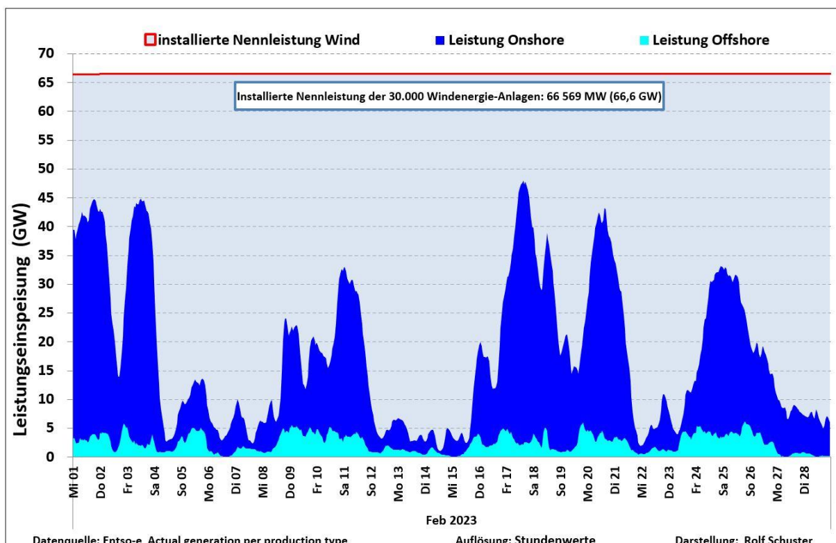
Abb. 1: Leistungsganglinie der Onshore/Offshore-Windenergie-Anlagen in Deutschland Febr 2023
