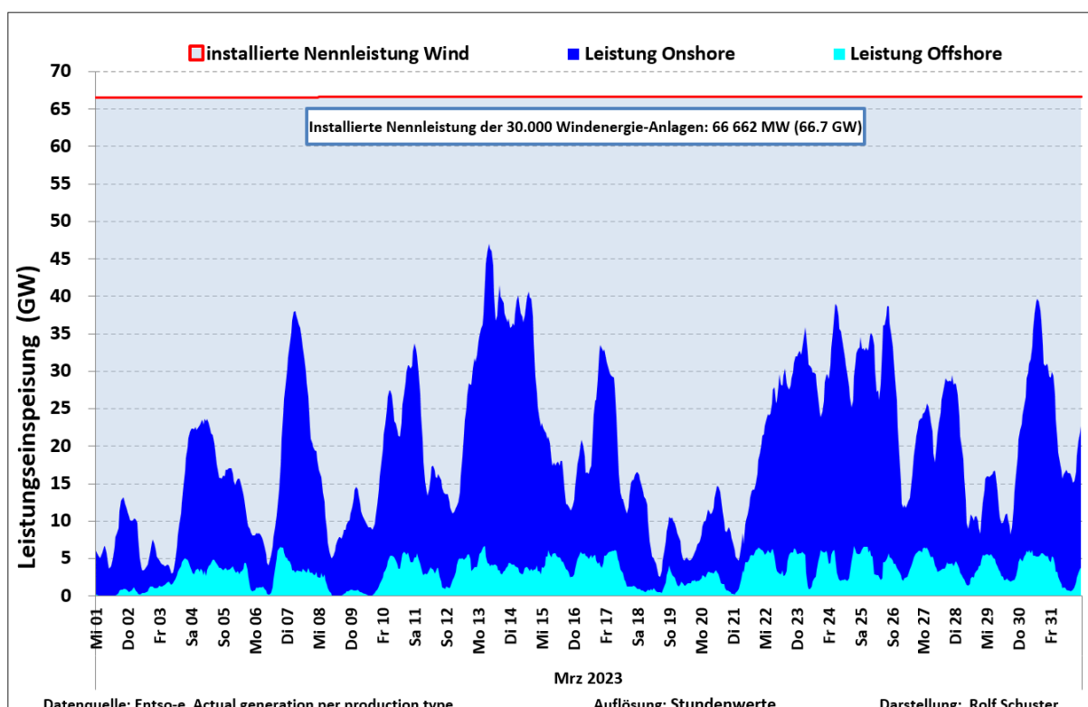
Abb. 1: Leistungsganglinie der Onshore/Offshore-Windenergie-Anlagen in Deutschland März 2023
