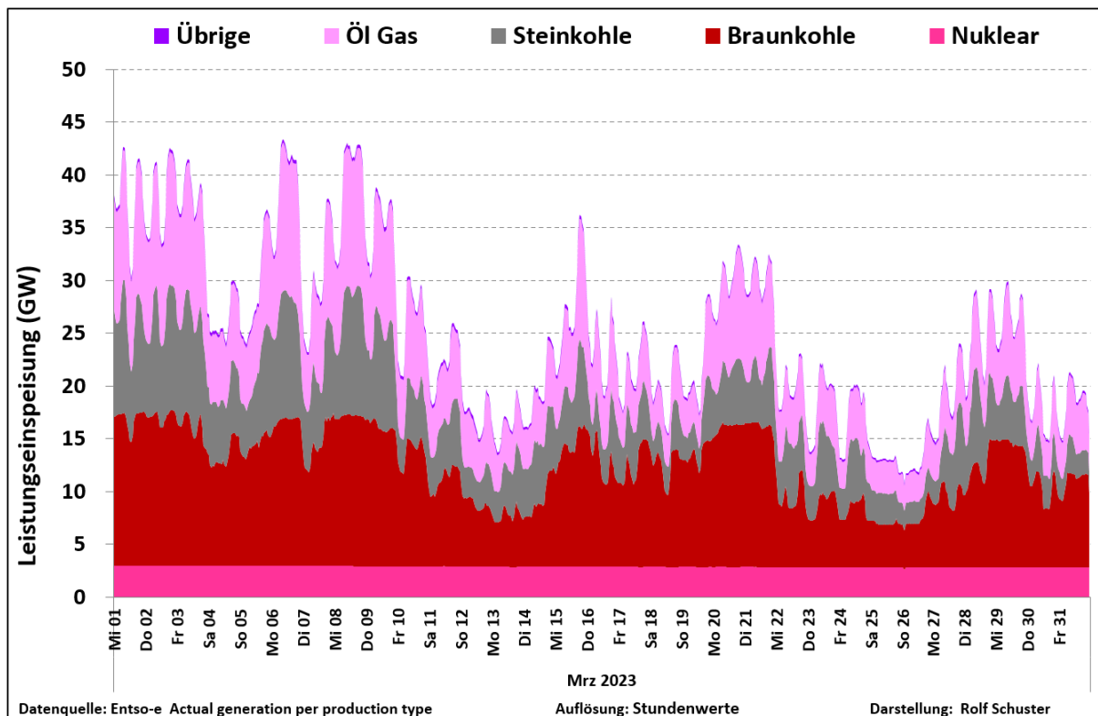
Abb. 4 Leistungsganglinien der konventionellen Anlagen Kohle, Öl, Gas und Kernenergie
