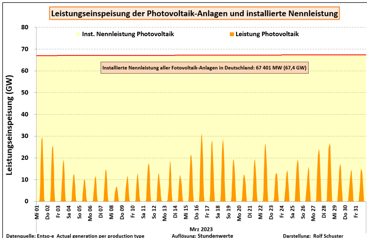
Abb. 2: Leistungsganglinie der Photovoltaik-Anlagen in Deutschland im März 2023
