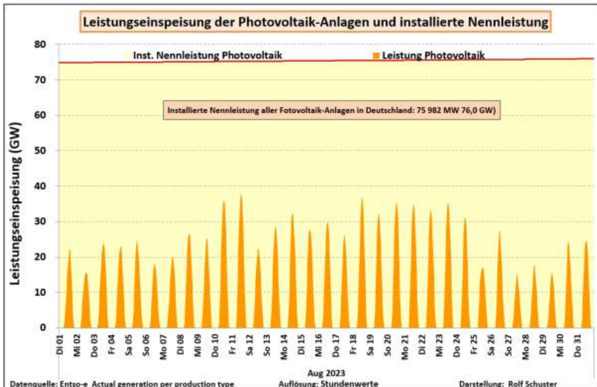
Abb. 2: Leistungsganglinie der Photovoltaik-Anlagen in Deutschland im August 2023
