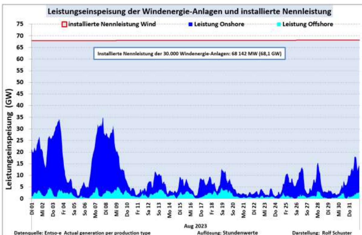
Abb. 1: Leistungsganglinie der Onshore/Offshore-Windenergie-Anlagen in Deutschland August 2023
