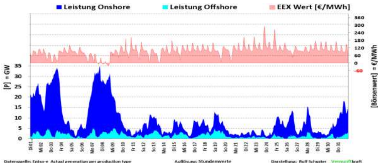
Abb. 8: Einspeisung Windenergie und Börsenpreise
