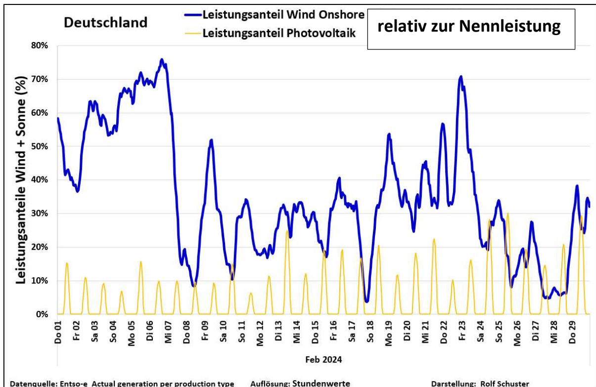
Abb. 5: Prozentuale Anteile der Erneuerbaren Energien Wind (Onshore) und Solar an der Leistungserzeugung im Februar 2024
