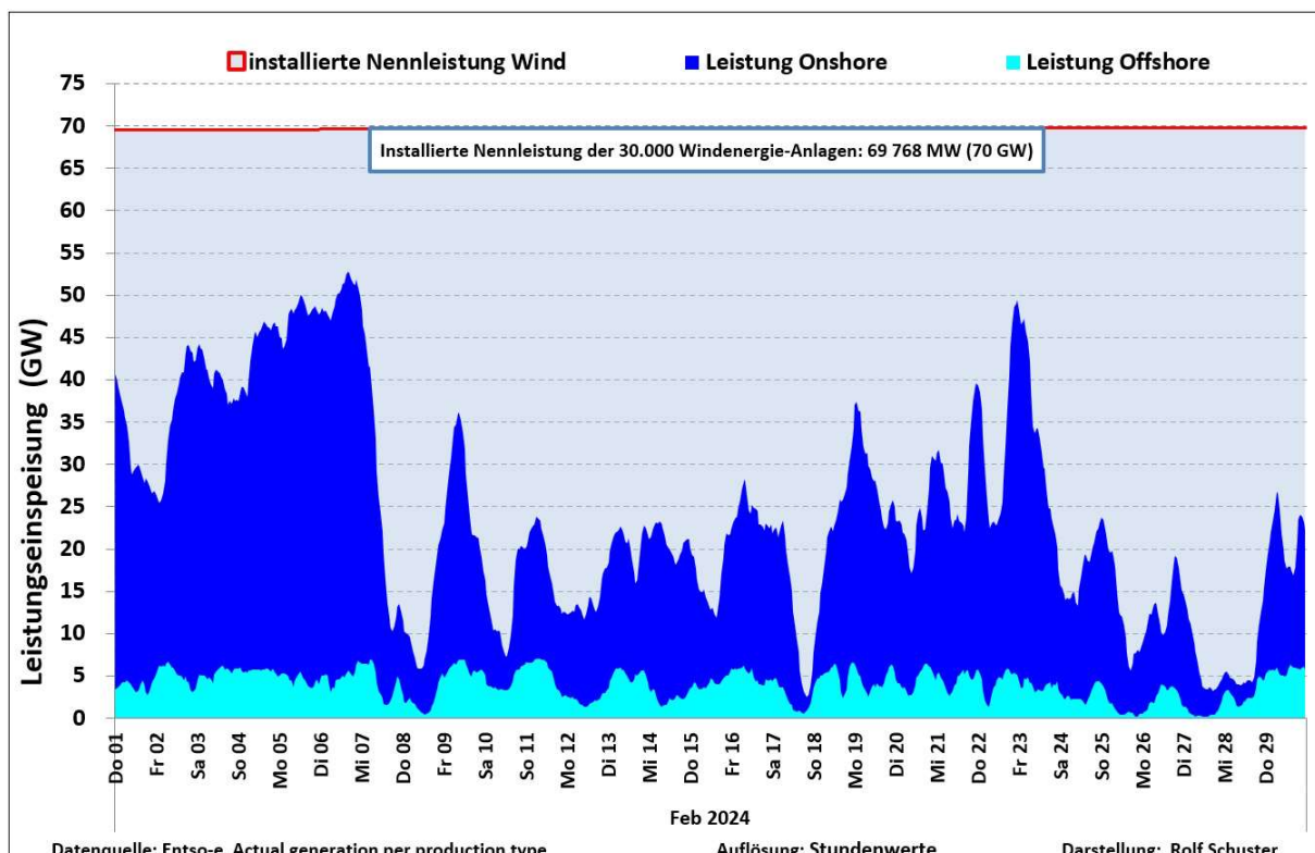
Abb. 1: Leistungsganglinie der Onshore/Offshore-Windenergie-Anlagen im Februar 2024
