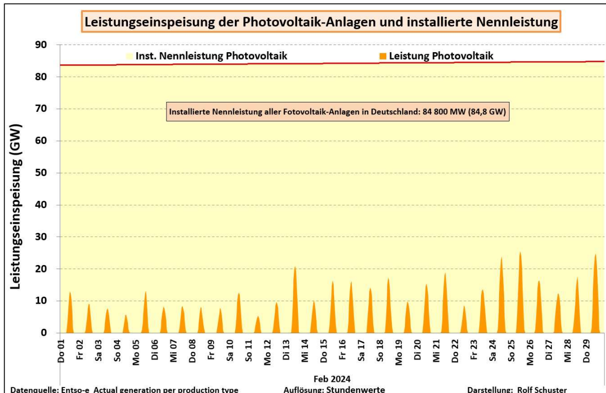
Abb. 2: Leistungsganglinie der Photovoltaik-Anlagen in Deutschland im Februar 2024
