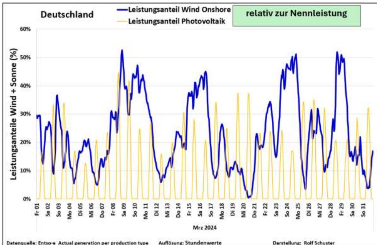
Abb. 5: Prozentuale Anteile der Erneuerbaren Energien Wind (Onshore) und Solar an der Leistungserzeugung im März 2024
