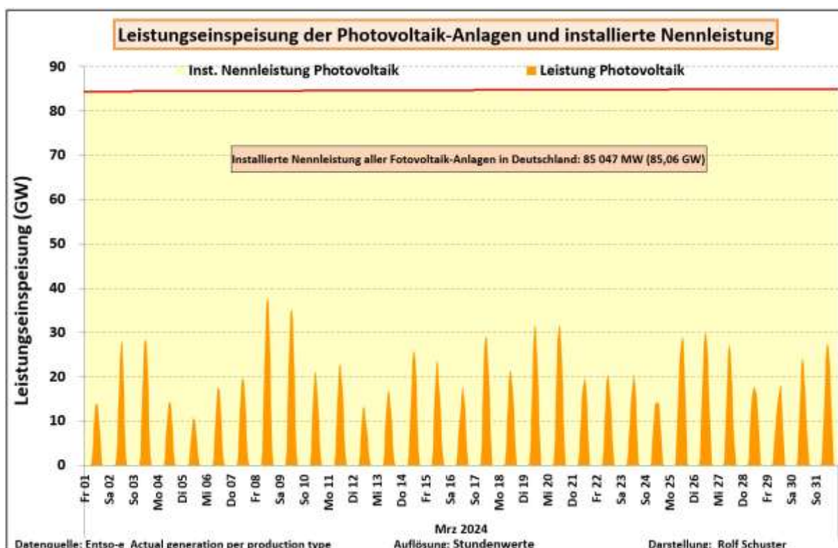
Abb. 2: Leistungsganglinie der Photovoltaik-Anlagen in Deutschland im März 2024
