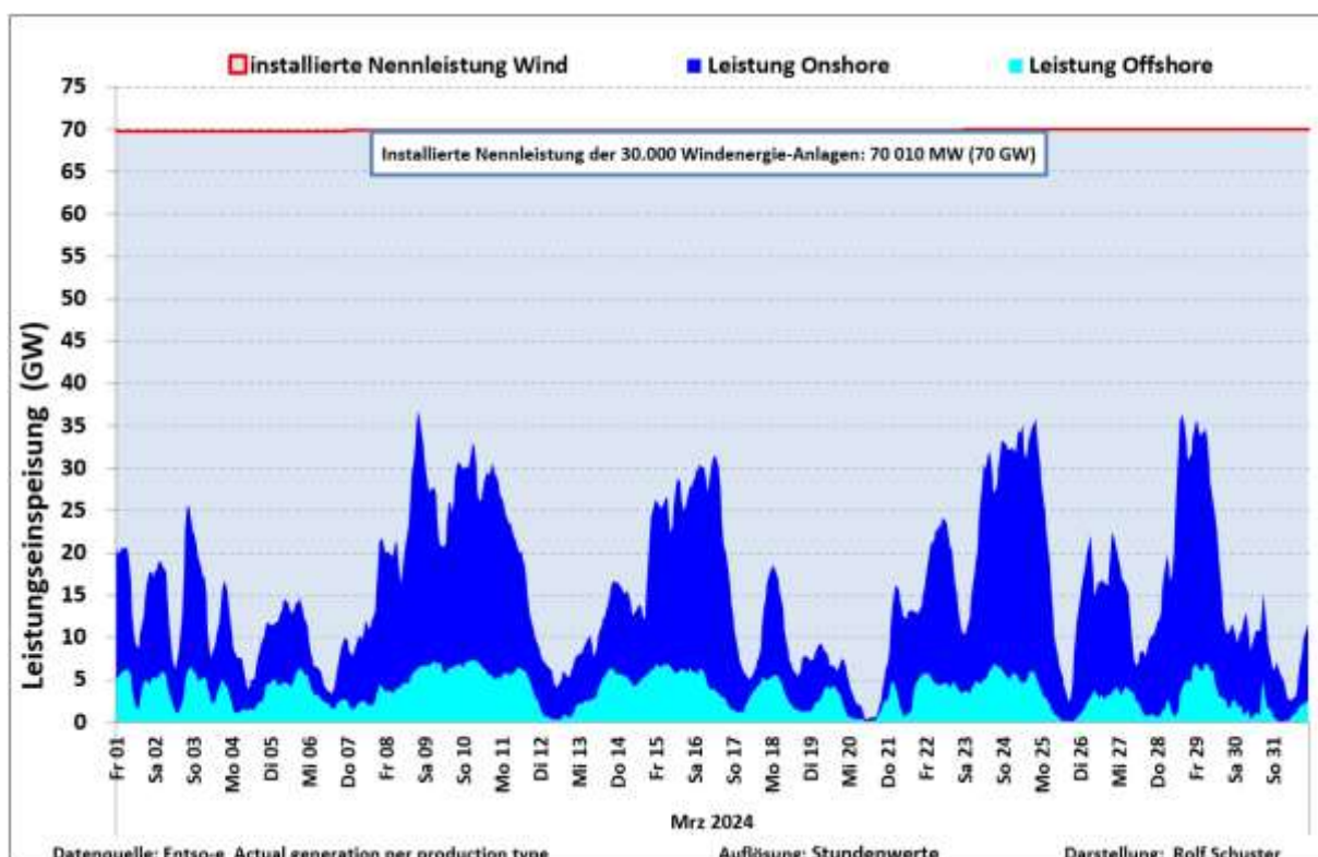
Abb. 1: Leistungsganglinie der Onshore/Offshore-Windenergie-Anlagen im März 2024
