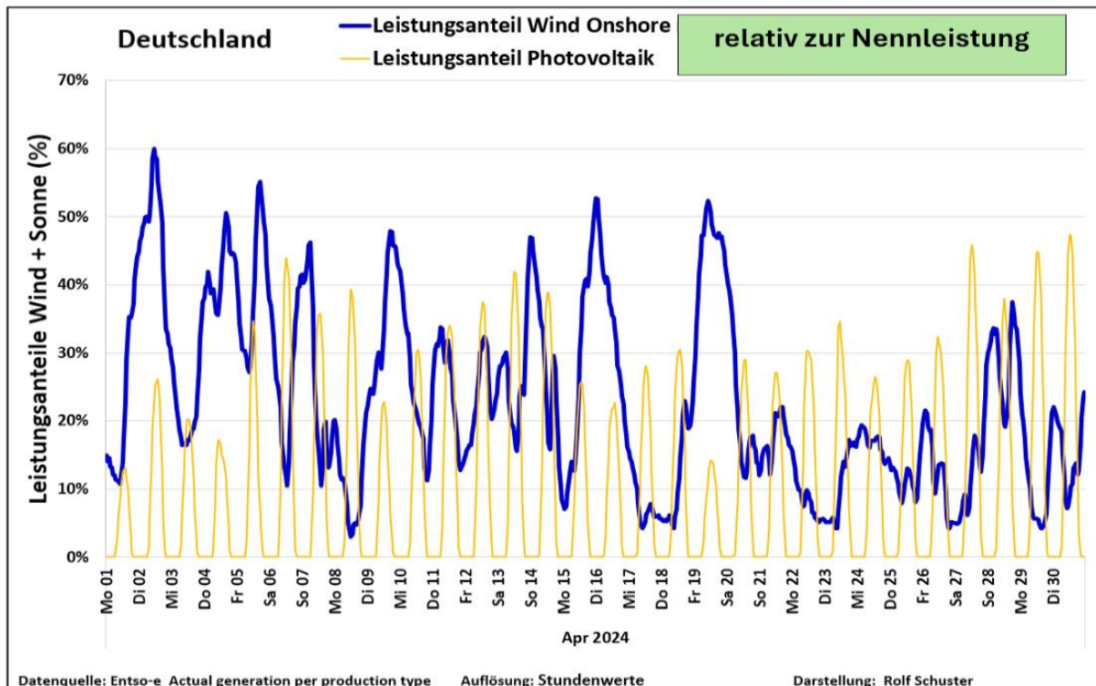
Abb. 5: Prozentuale Anteile der Erneuerbaren Energien Wind (Onshore) und Solar an der Leistungserzeugung im April 2024
