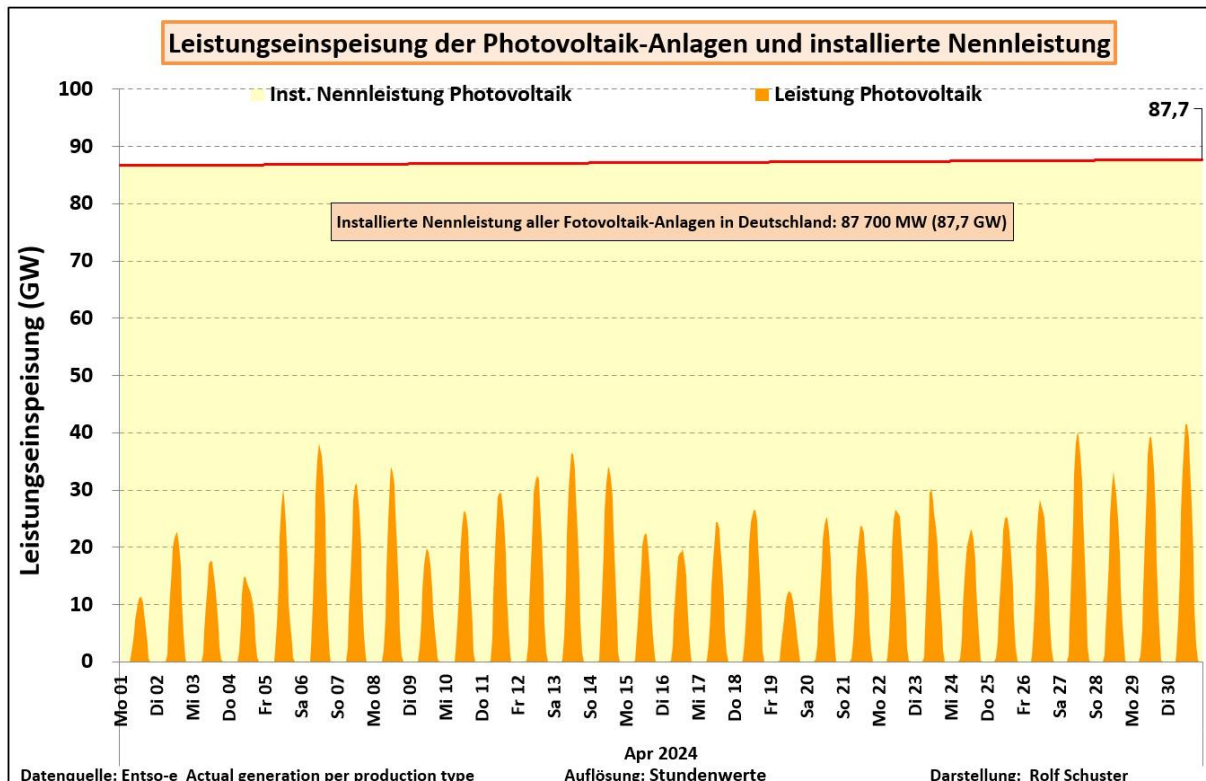
Abb. 2: Leistungsganglinie der Photovoltaik-Anlagen in Deutschland im April 2024
