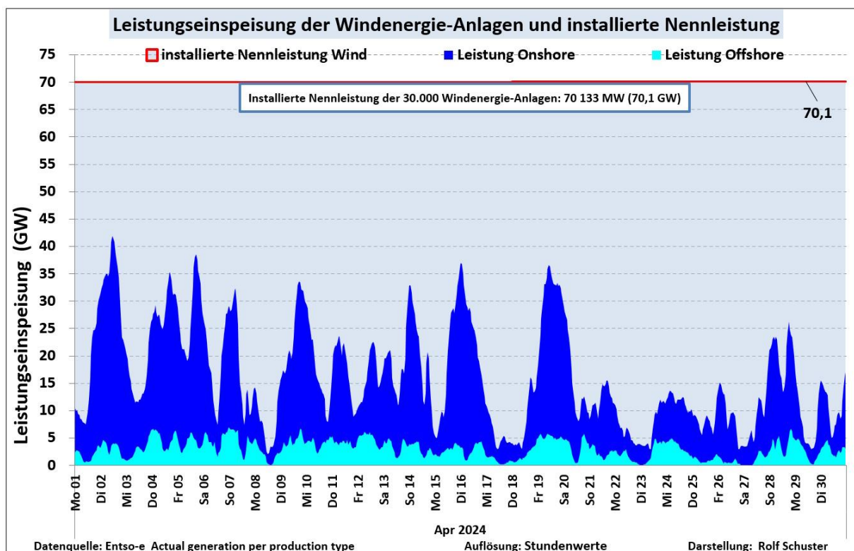
Abb. 1: Leistungsganglinie der Onshore/Offshore-Windenergie-Anlagen im April 2024
