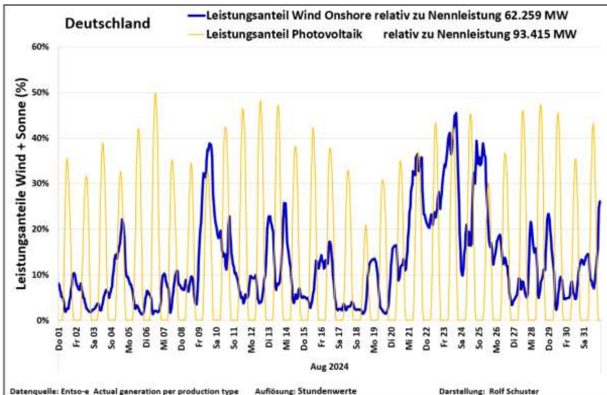
Abb. 5: Prozentuale Anteile EE Wind (Onshore) und Solar an der Leistungserzeugung im August 2024
