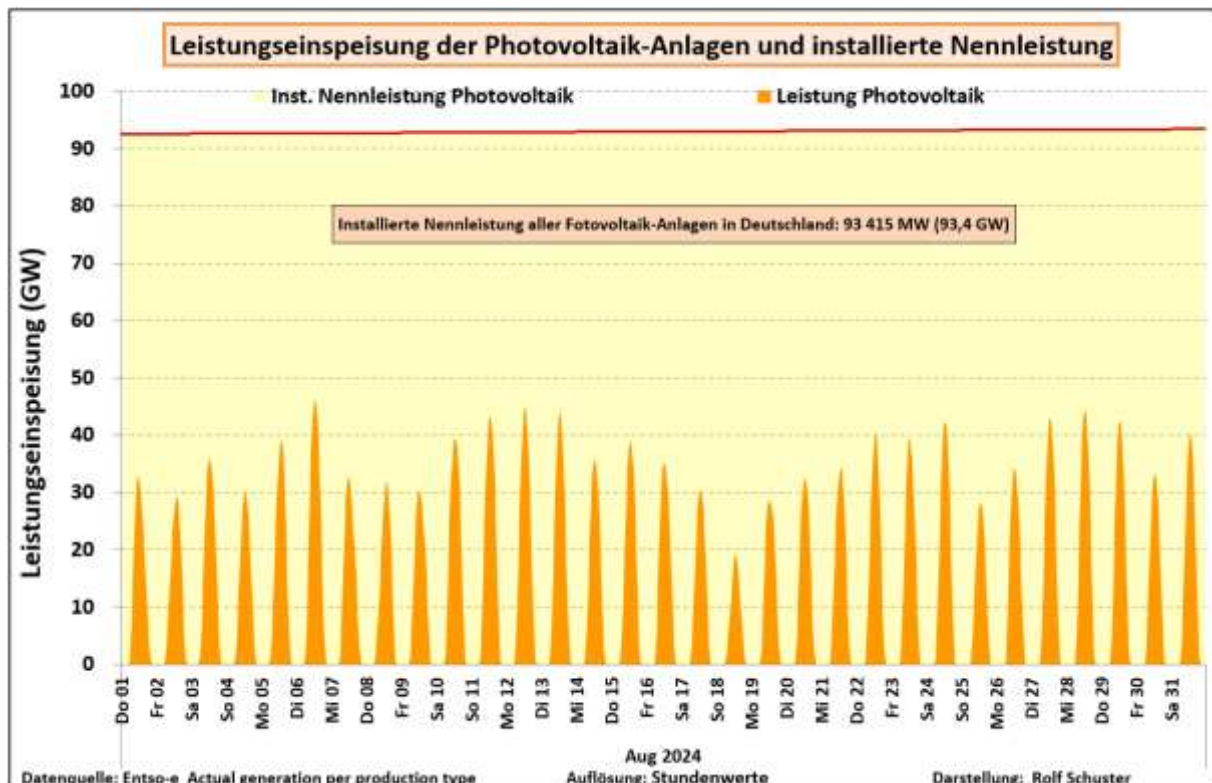
Abb. 2: Leistungsganglinie der Photovoltaik-Anlagen in Deutschland im August 2024
