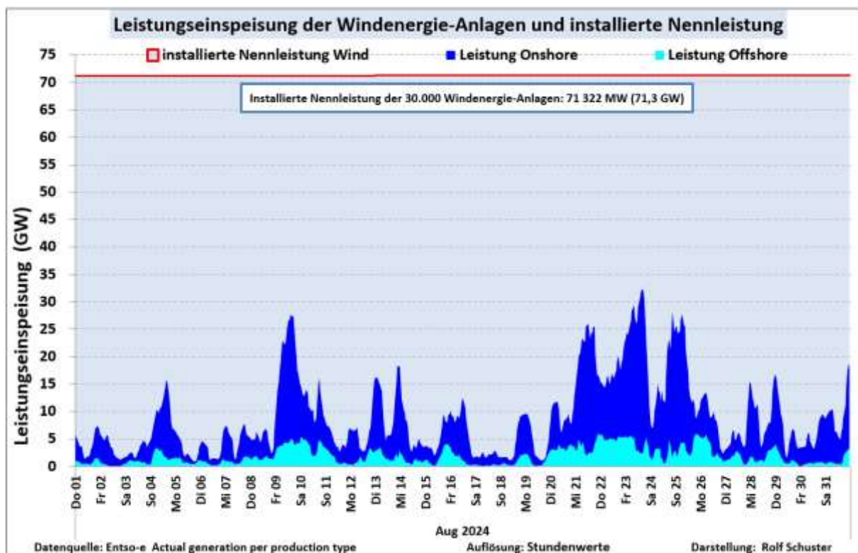
Abb. 1: Leistungsganglinie der Onshore/Offshore-Windenergie-Anlagen im August 2024
