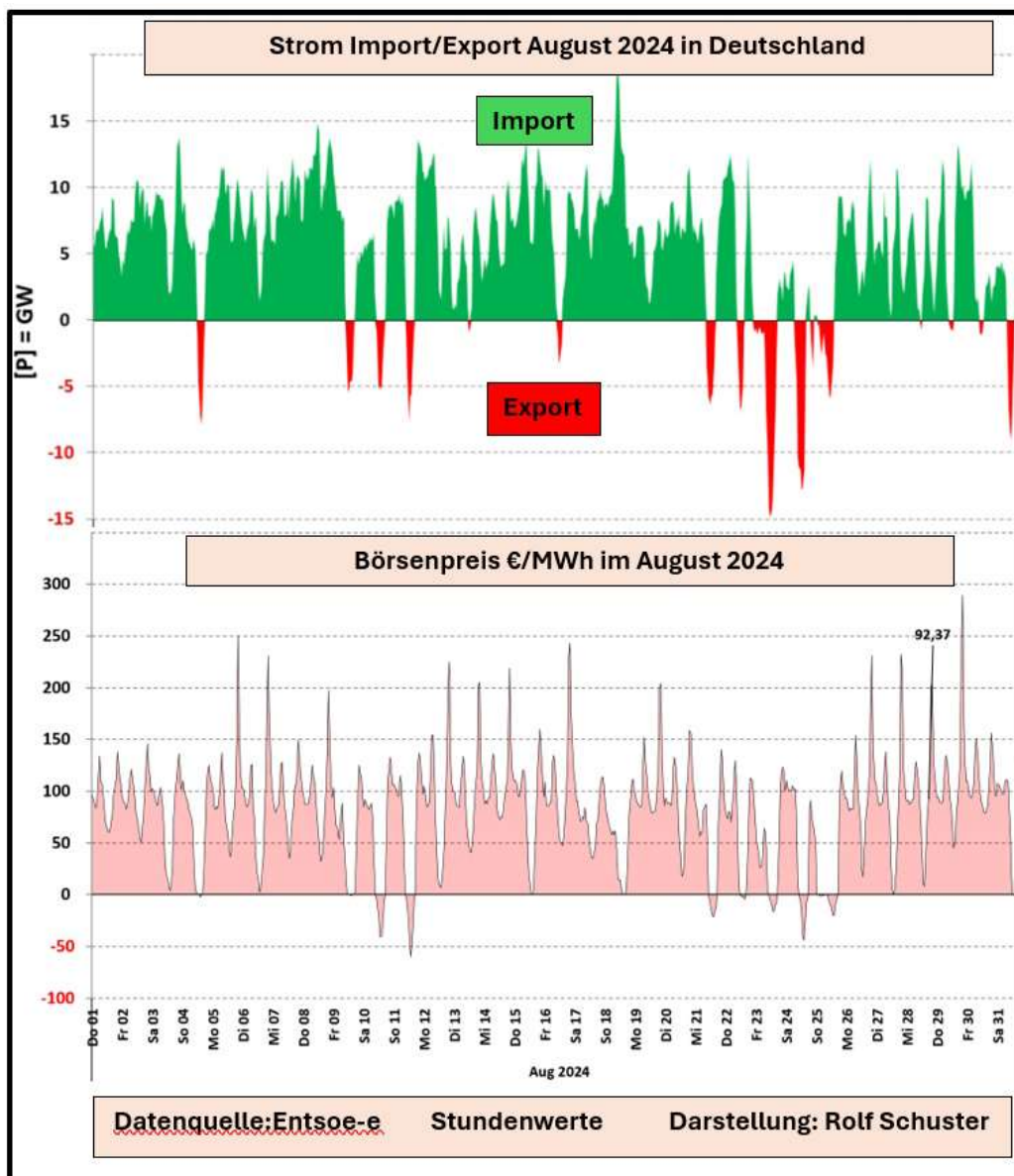
Abb. 7: Strom-Export/Import und Börsenentwicklung
