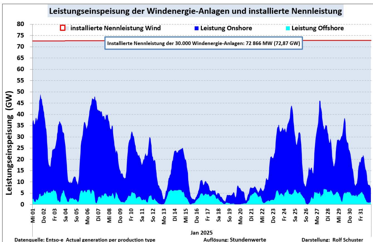
Abb. 1: Leistungsganglinie der Onshore/Offshore-Windenergie-Anlagen im Januar 2025
