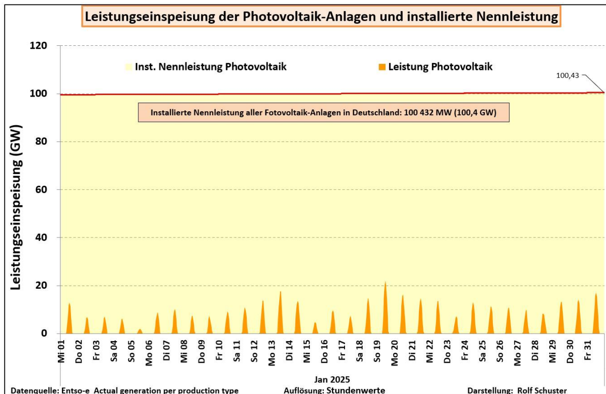
Abb. 2: Leistungsganglinie der Photovoltaik-Anlagen in Deutschland im Januar 2025
