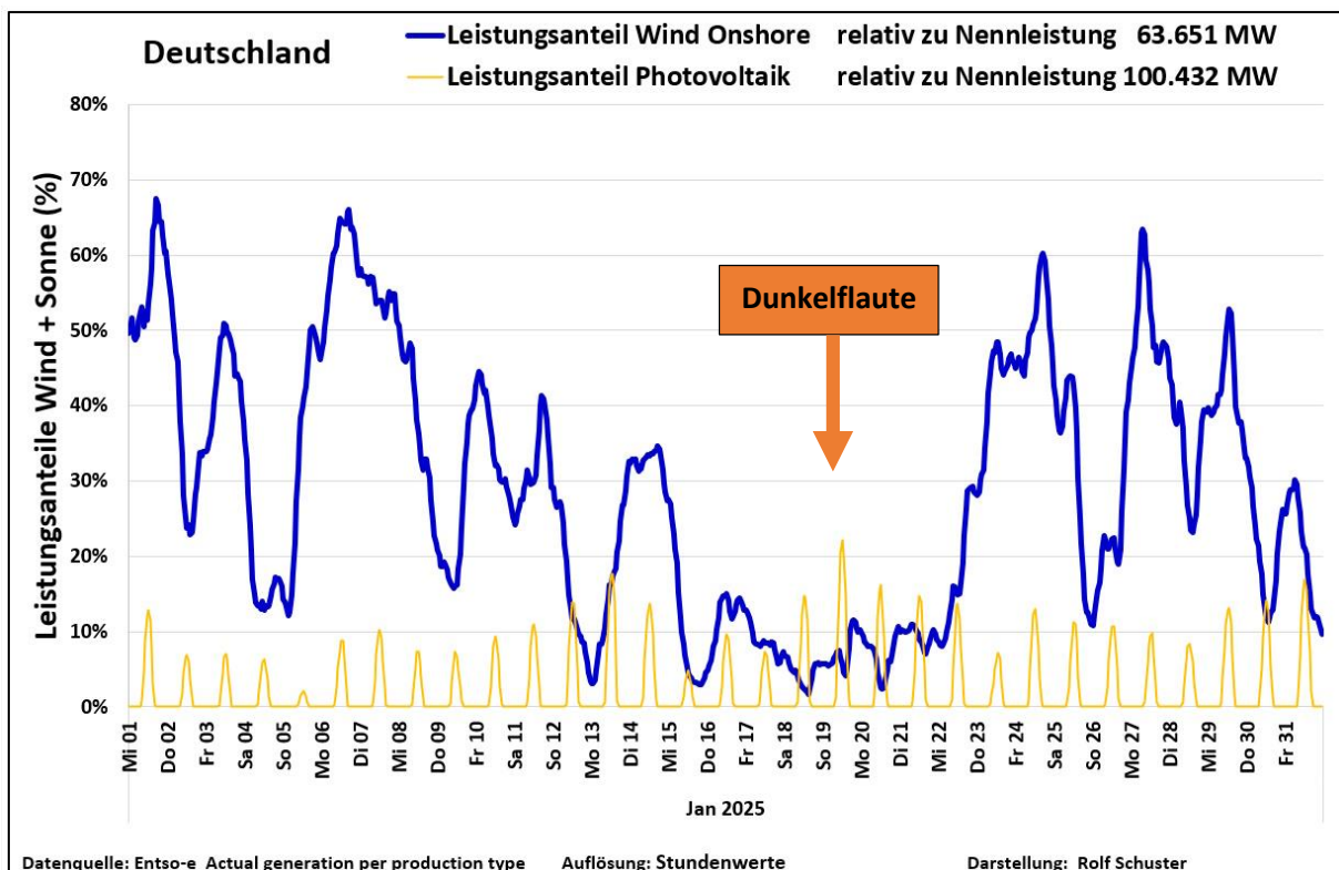
Abb. 5: Prozentuale Anteile EE Wind (Onshore) und Solar an der Leistungserzeugung im Jan. 2025
