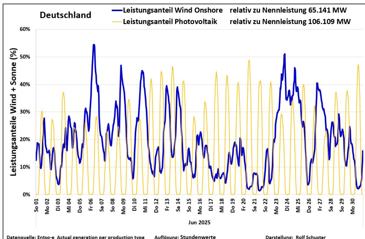
Abb. 5: Prozentuale Anteile EE Wind (Onshore) und Solar an der Leistungserzeugung im Juni 2025
