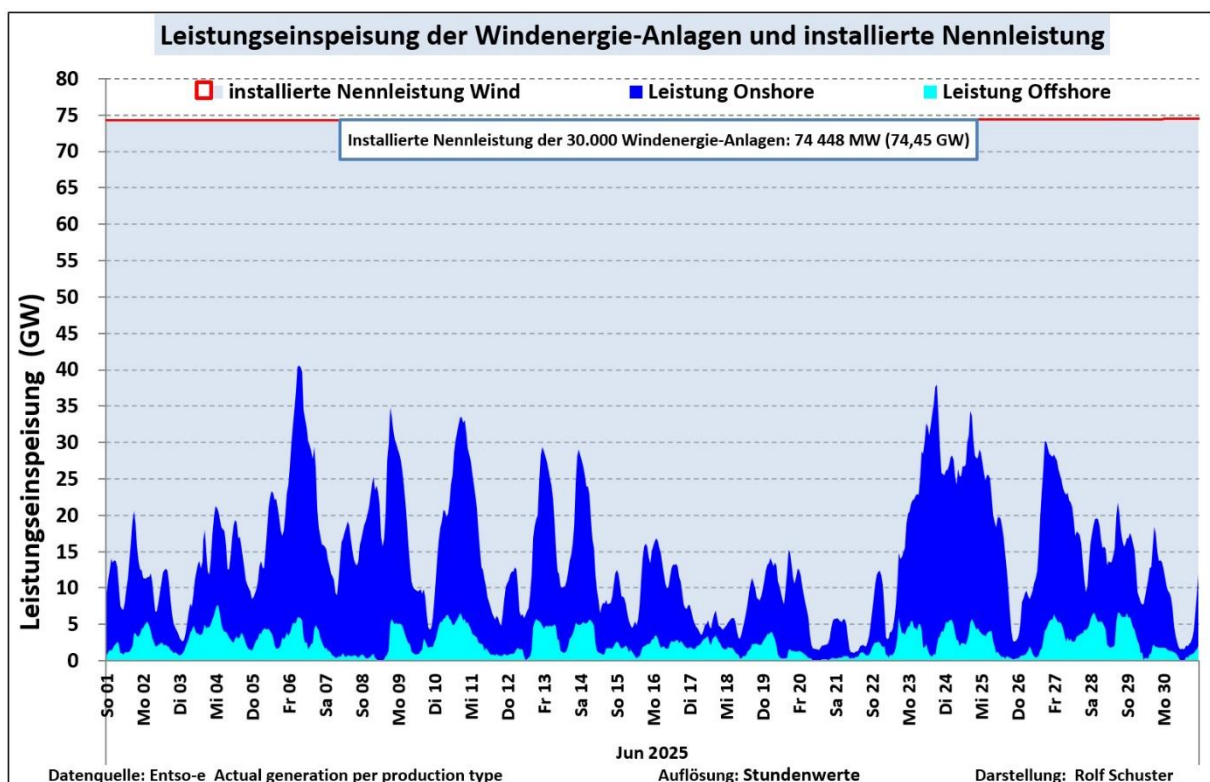
Abb. 1: Leistungsganglinie der Onshore/Offshore-Windenergie-Anlagen im Juni 2025
