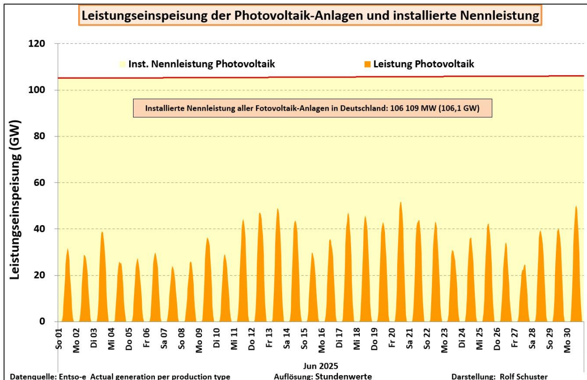
Abb. 2: Leistungsganglinie der Photovoltaik-Anlagen in Deutschland im Juni 2025
