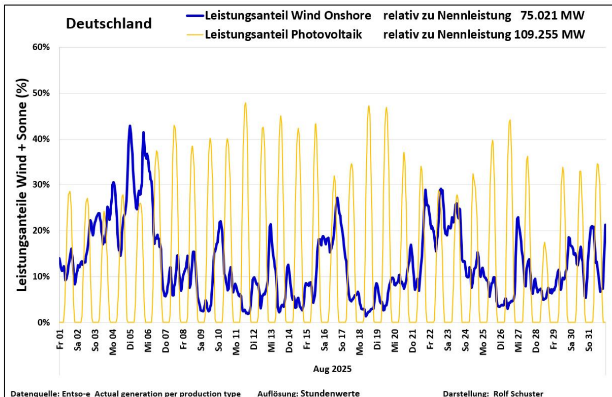
Abb. 5: Prozentuale Anteile EE Wind (Onshore) und Solar an der Leistungserzeugung im August 2025
