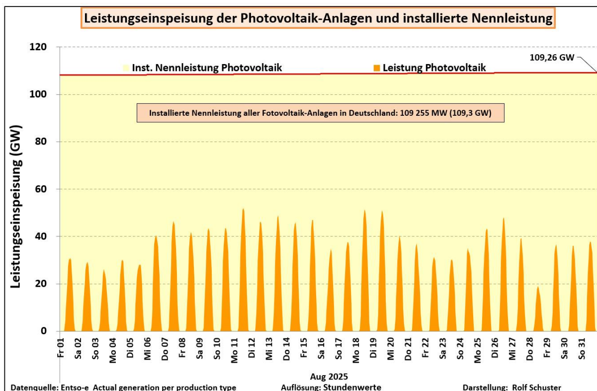
Abb. 2: Leistungsganglinie der Photovoltaik-Anlagen in Deutschland im August 2025
