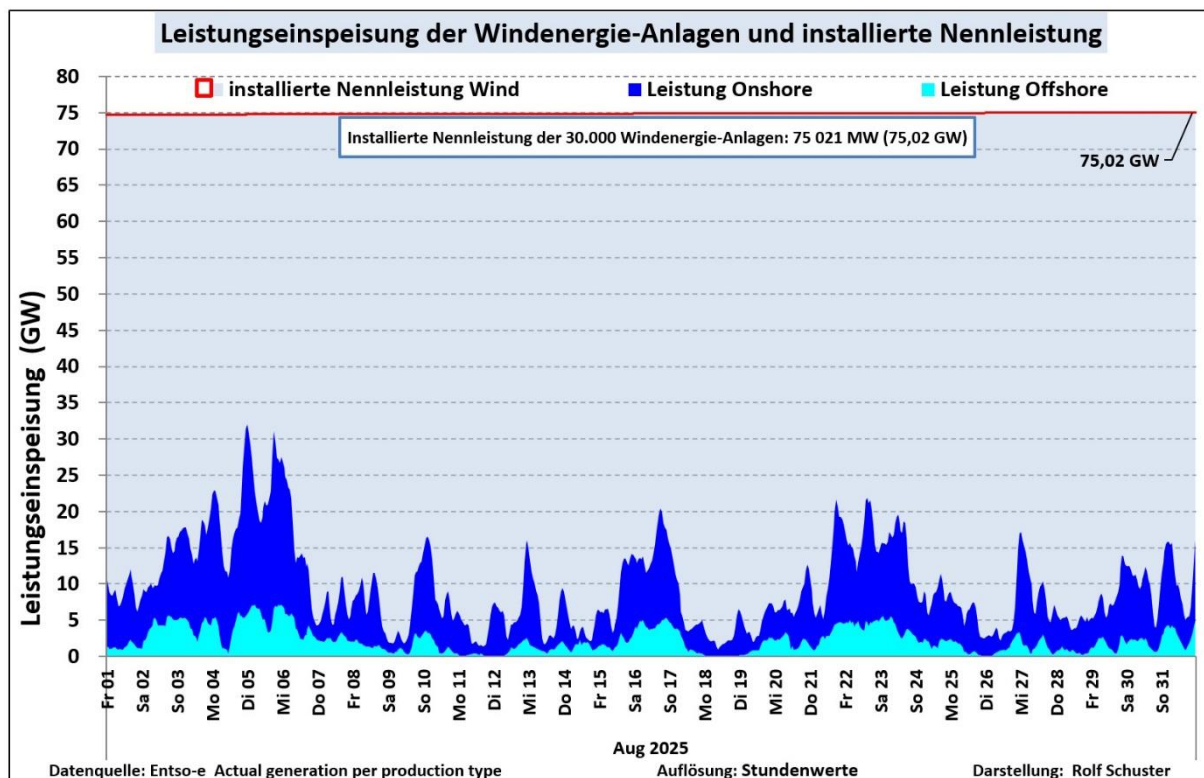
Abb. 1: Leistungsganglinie der Onshore/Offshore-Windenergie-Anlagen im August 2025
