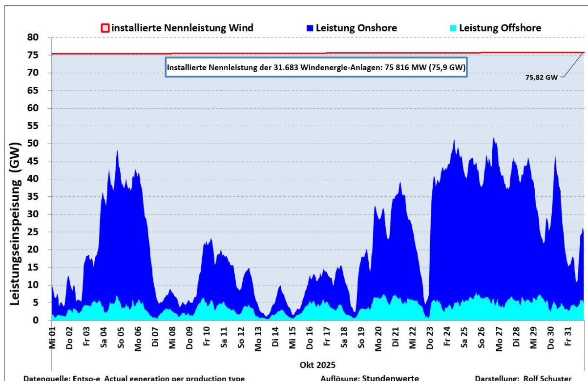
Abb. 1: Leistungsganglinie der Onshore/Offshore-Windenergie-Anlagen im Oktober 2025
