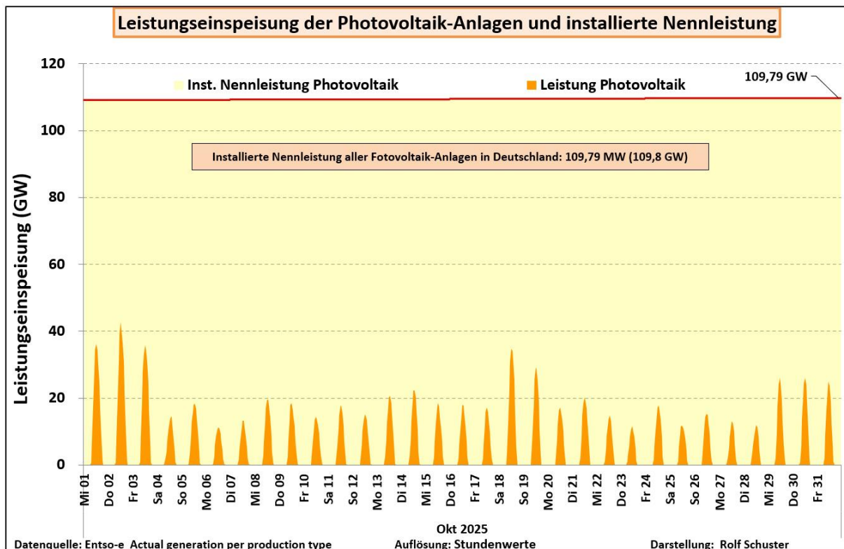
Abb. 2: Leistungsganglinie der Photovoltaik-Anlagen in Deutschland im Oktober 2025
