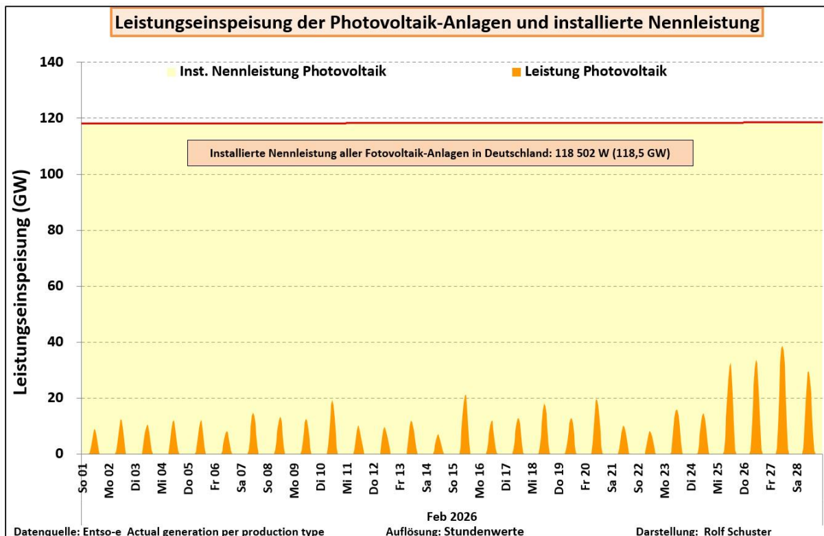
Abb. 2: Leistungsganglinie der Photovoltaik-Anlagen in Deutschland im Februar 2026
