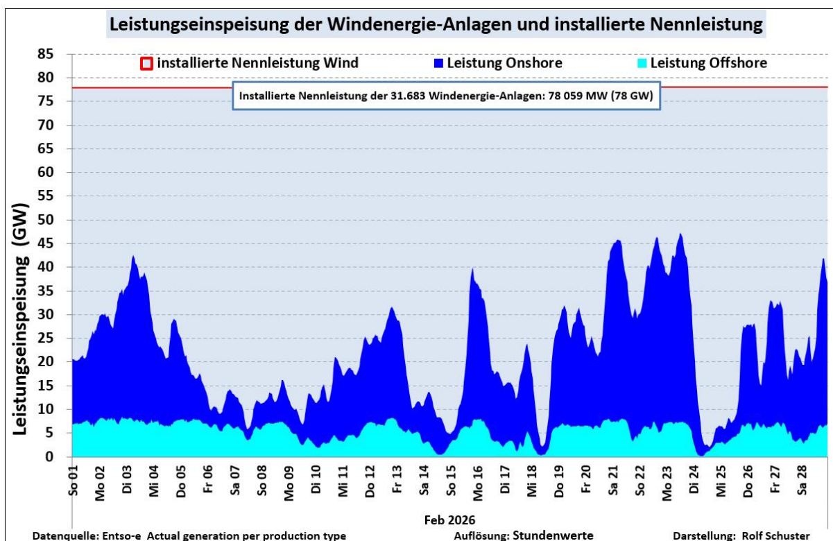
Abb. 1: Leistungsganglinie der Onshore/Offshore-Windenergie-Anlagen im Februar 2026
