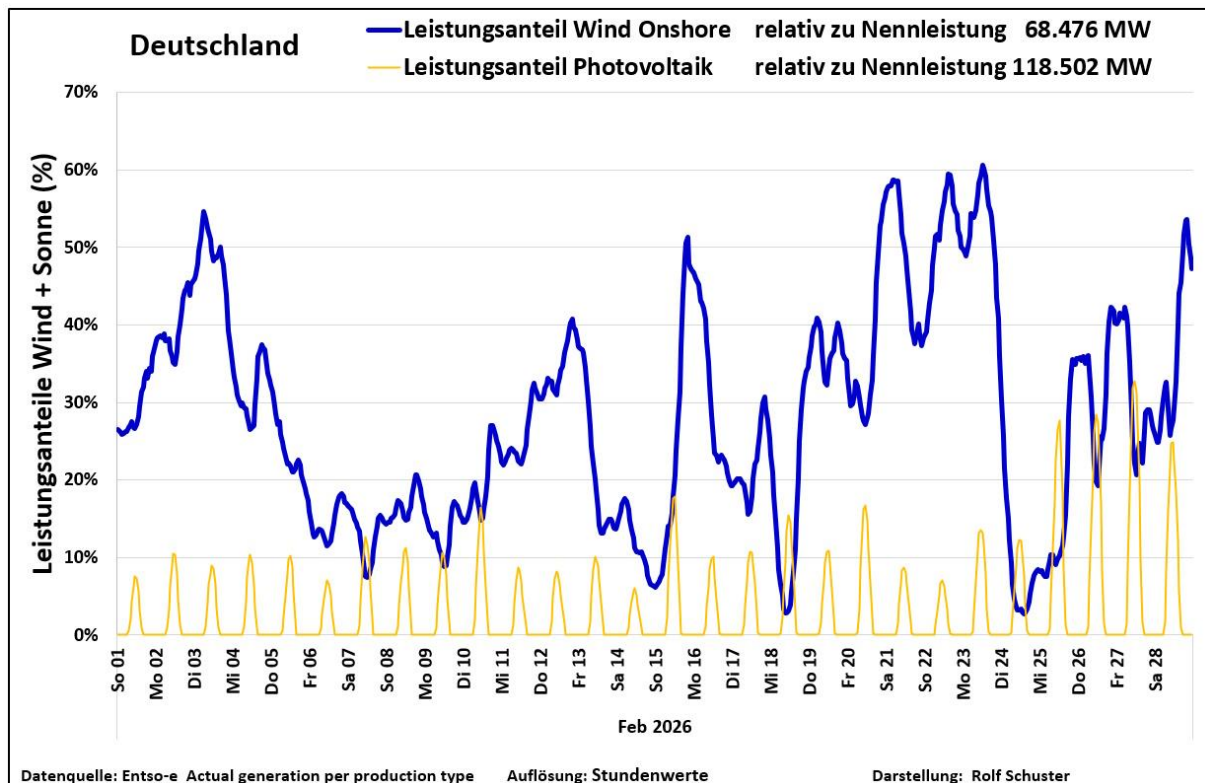
Abb. 5: Prozentuale Anteile EE Wind (Onshore) und Solar an der Leistungserzeugung im Febr 2026
