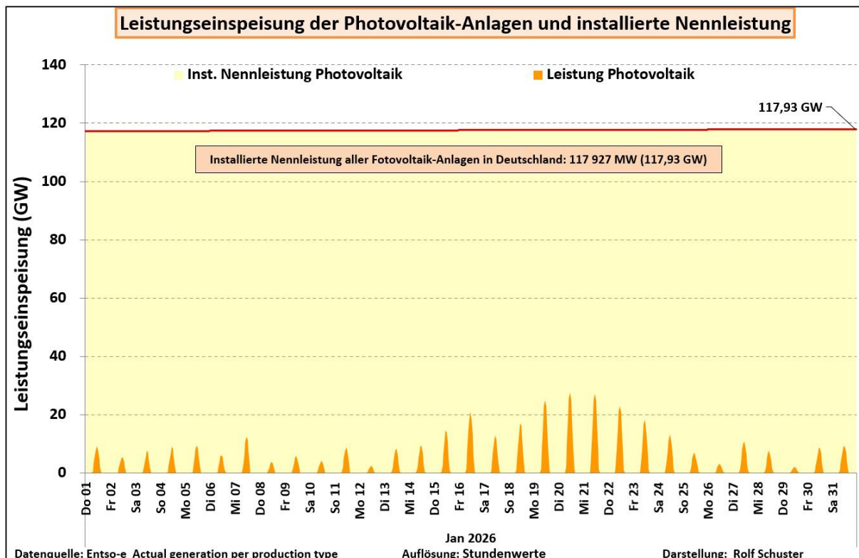
Abb. 2: Leistungsganglinie der Photovoltaik-Anlagen in Deutschland im Januar 2026
