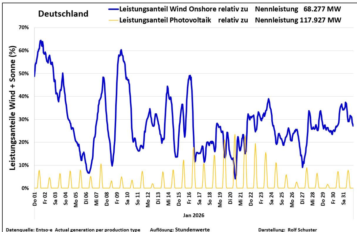
Abb. 5: Prozentuale Anteile EE Wind (Onshore) und Solar an der Leistungserzeugung im Jan 2026
