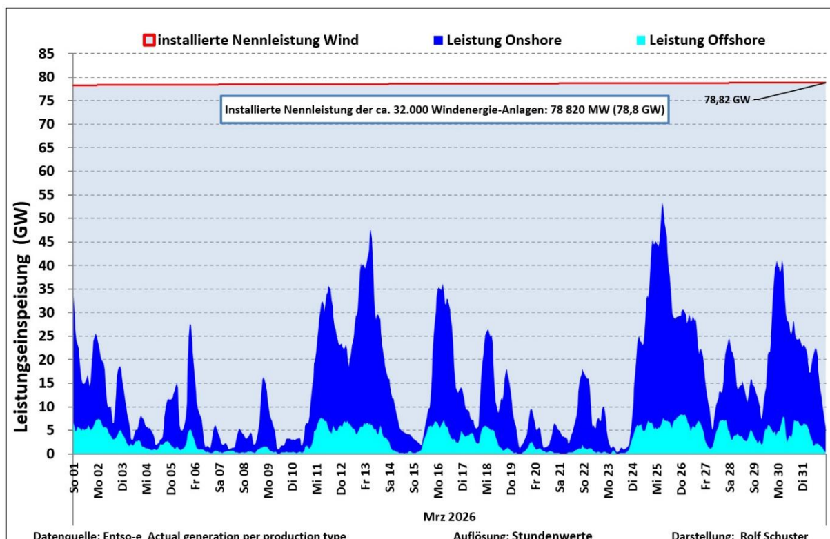
Abb. 1: Leistungsganglinie der Onshore/Offshore-Windenergie-Anlagen im März 2026
