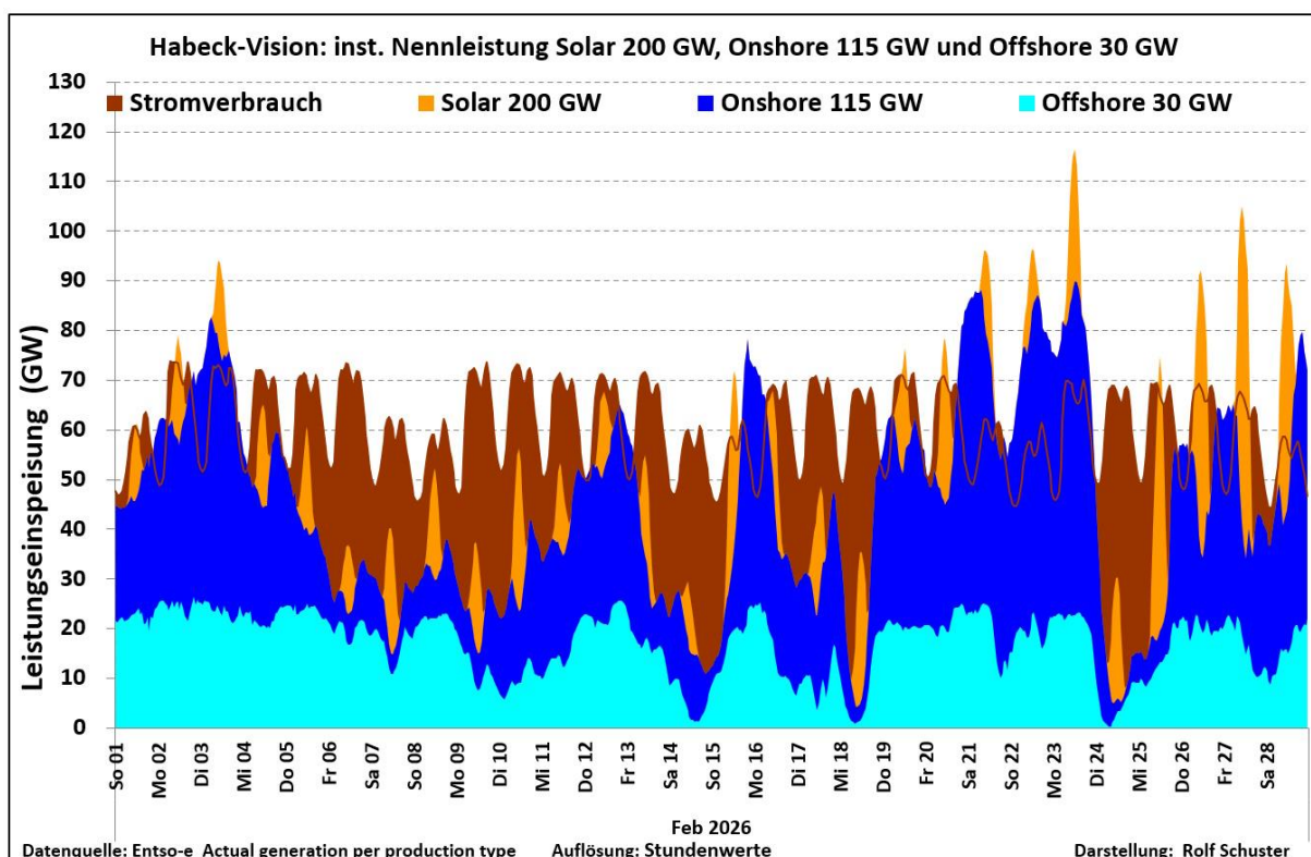
Abb. 6: Habeck-Vision (Ausbau der installierten Nennleistungen Windenergie auf 145.000 MW und Solar auf 200.00 MW); Leistungseinspeisung Wind+Solar auf diese Nennleistungen hochskaliert.
