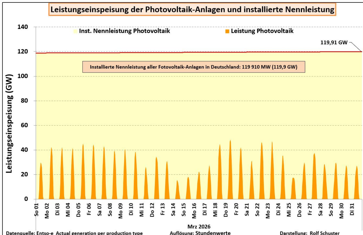
Abb. 2: Leistungsganglinie der Photovoltaik-Anlagen in Deutschland im März 2026
