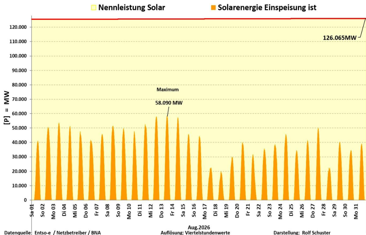
Abb. 2: Leistungsganglinie der Photovoltaik-Anlagen in Deutschland im August 2026
