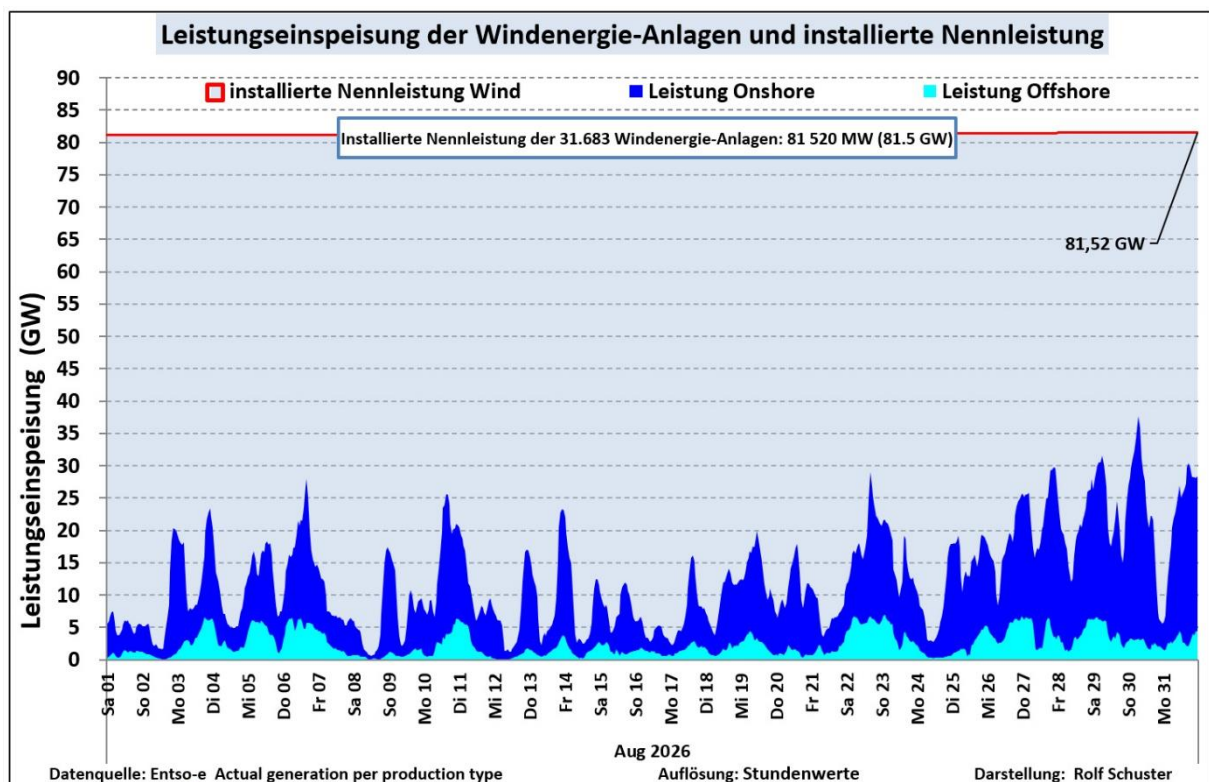
Abb. 1: Leistungsganglinie der Onshore/Offshore-Windenergie-Anlagen im August 2026
