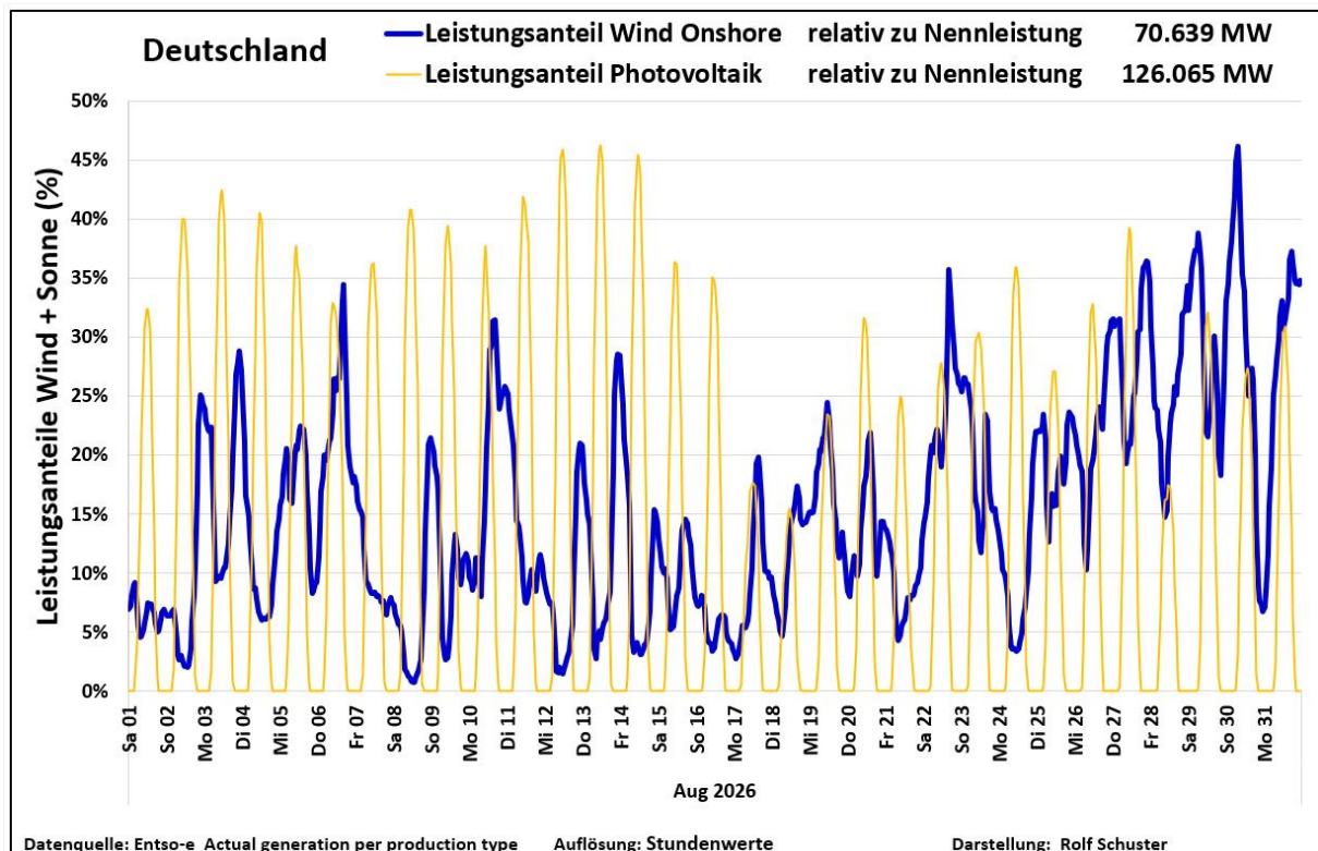
Abb. 5: Prozentuale Anteile EE Wind (Onshore) und Solar an der Leistungserzeugung im August 2026
